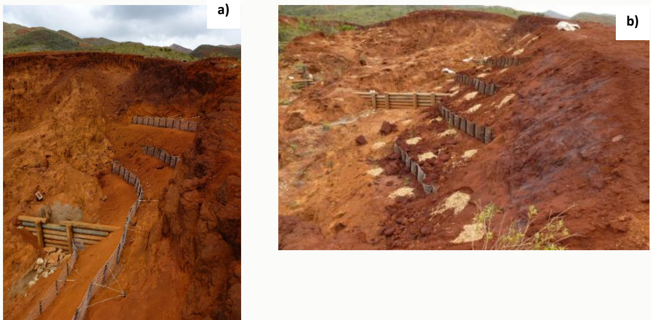
Figure 32. Exemple de travaux de terrassement et d'écarterement des berges et des talus
