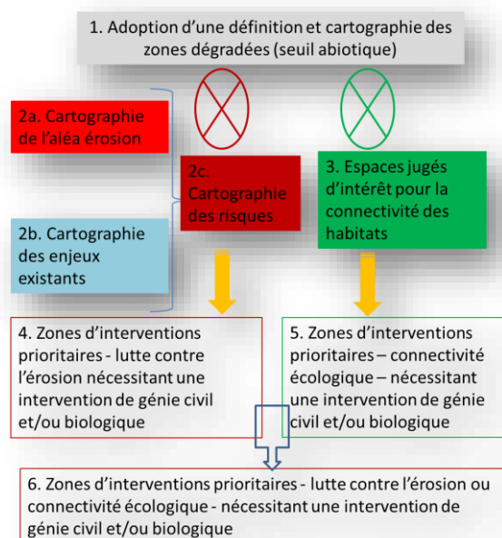
Figure 17. schéma de l'approche méthodologique globale utilisée pour l'identification des zones d'interventions prioritaires.
